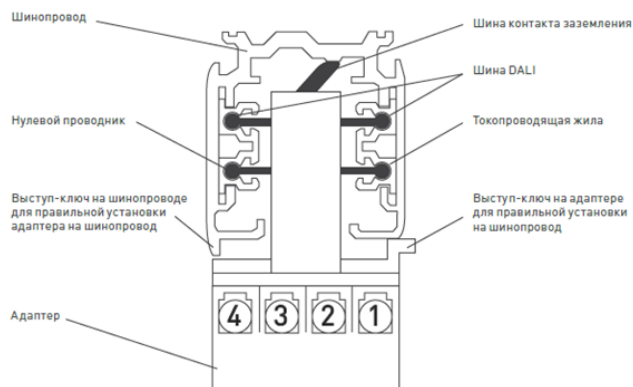
Рисунок 1. Подключение адаптера к шинопроводу
